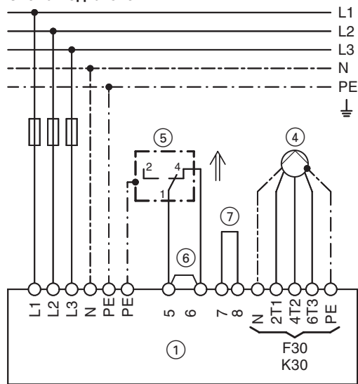
Схема подключения
