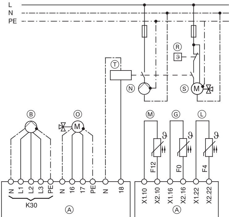
Схема подключения
