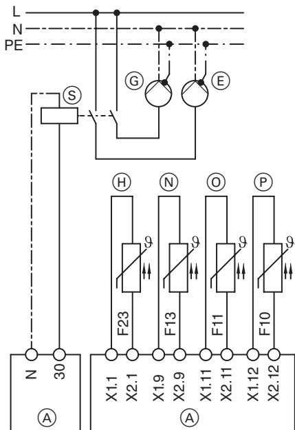
Схема подключения
