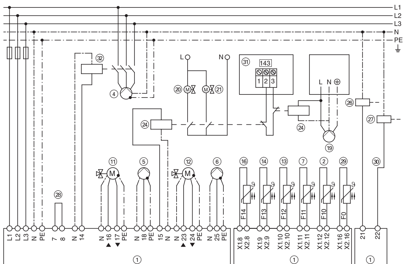
Схема подключения устройства управления 1-м. подчиненным тепловым насосом
