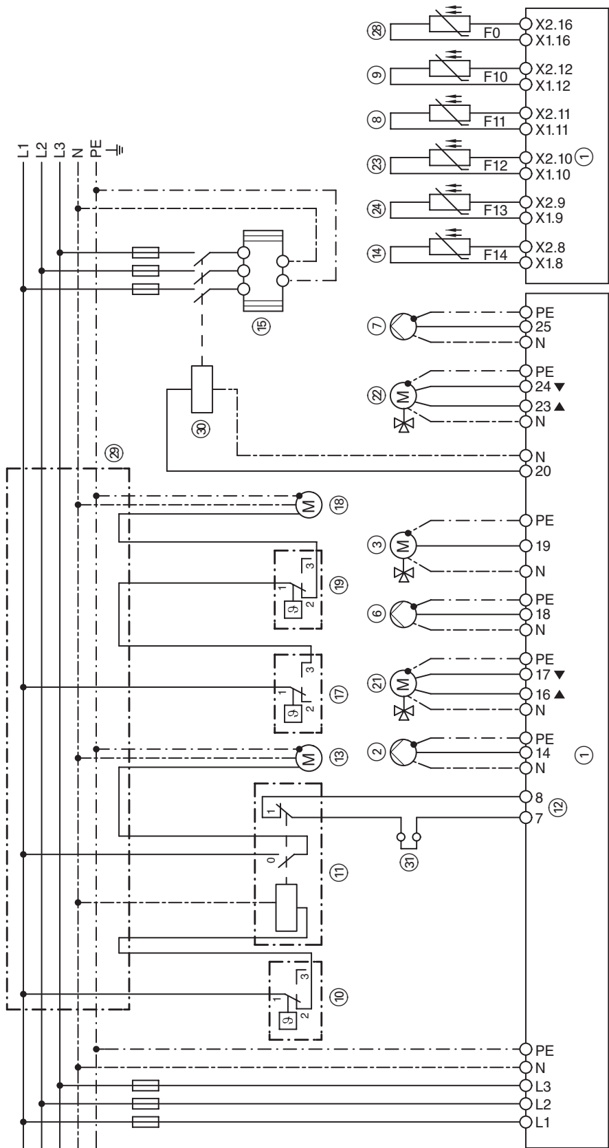
Схема подключения
