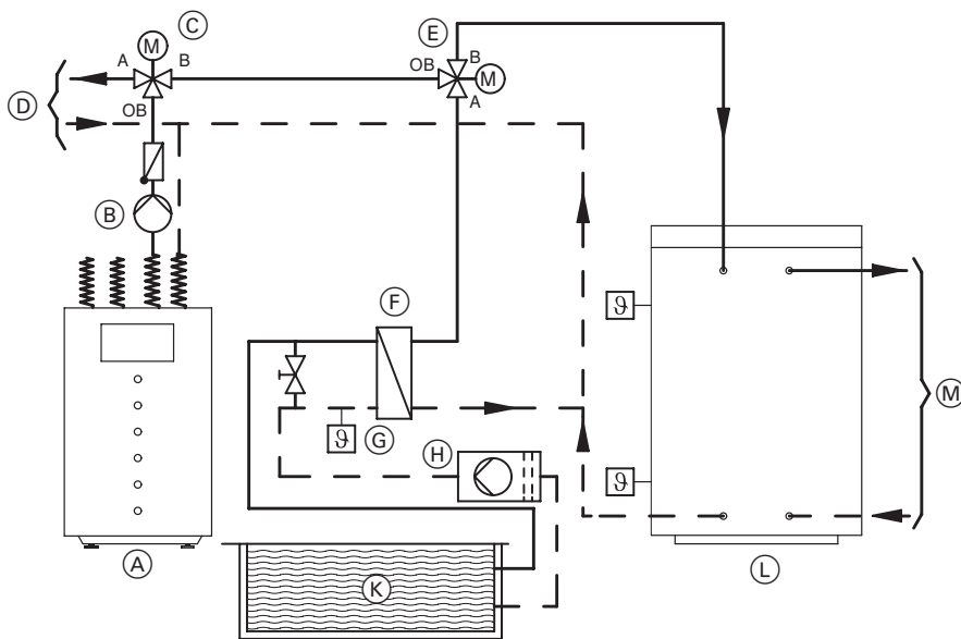
Схема подключения
