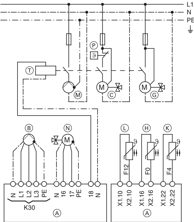
Схема подключения
