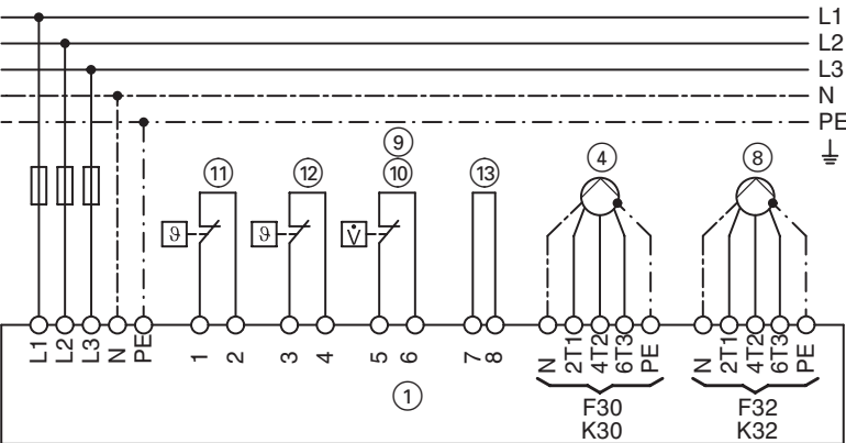
Схема подключения
