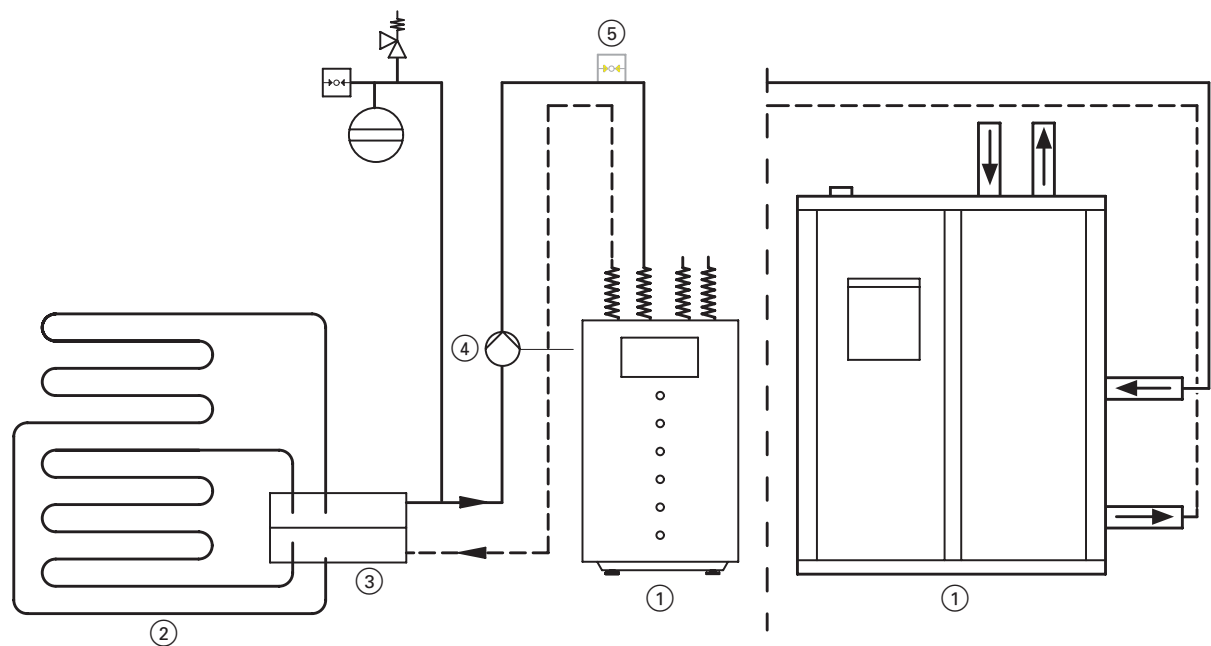
Схема подключения
