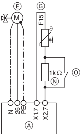
Схема подключения
