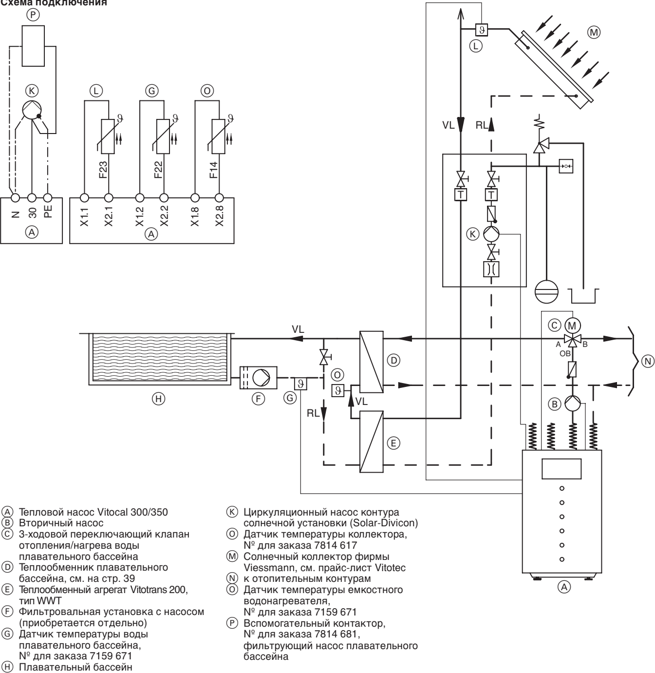
Схема подключения
