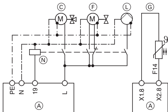
Схема подключения
