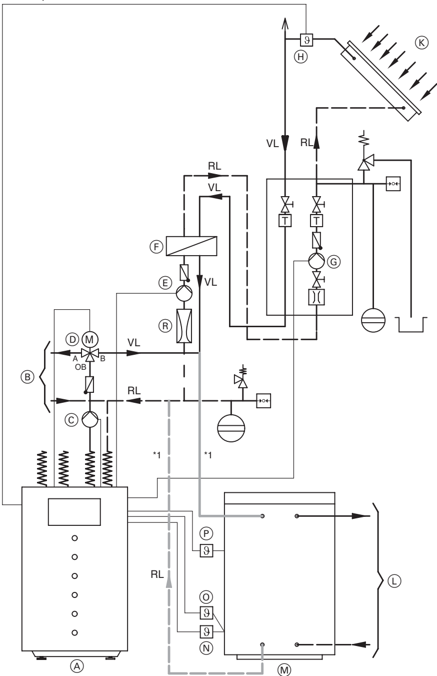
Схема подключения
