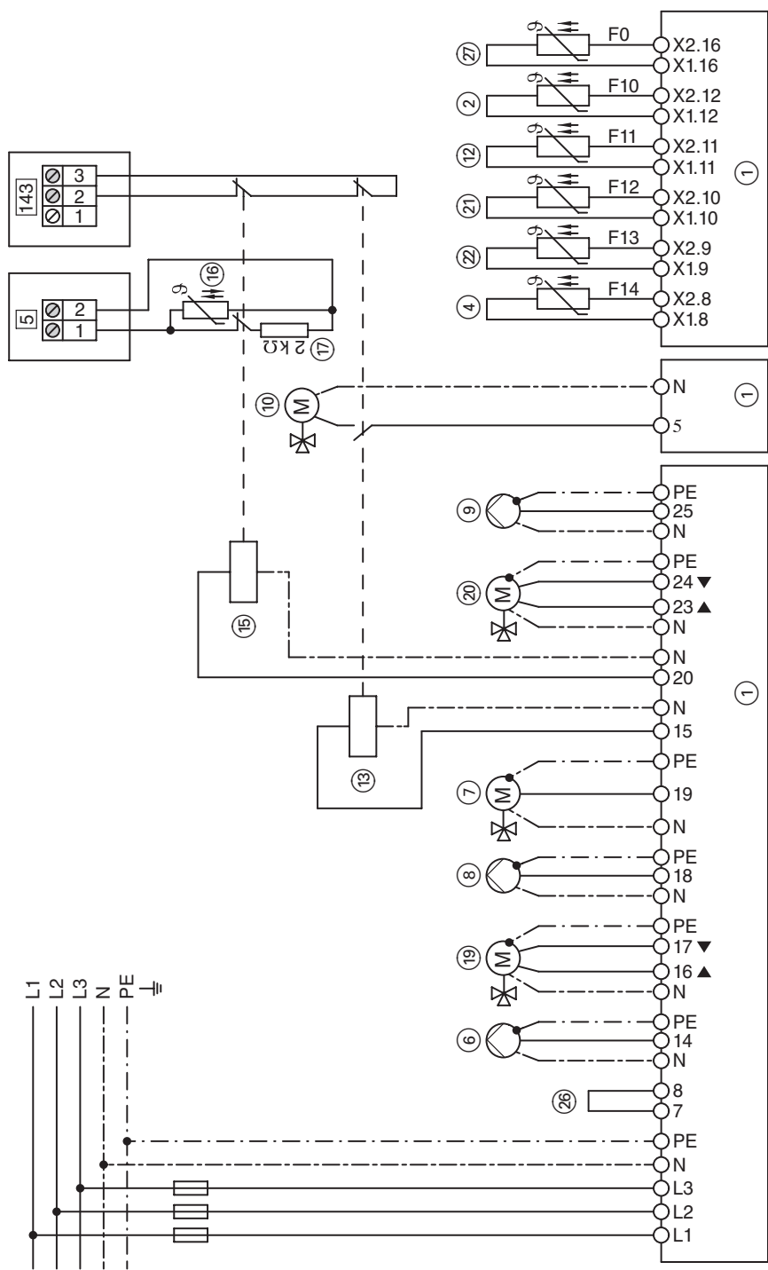
Схема подключения
