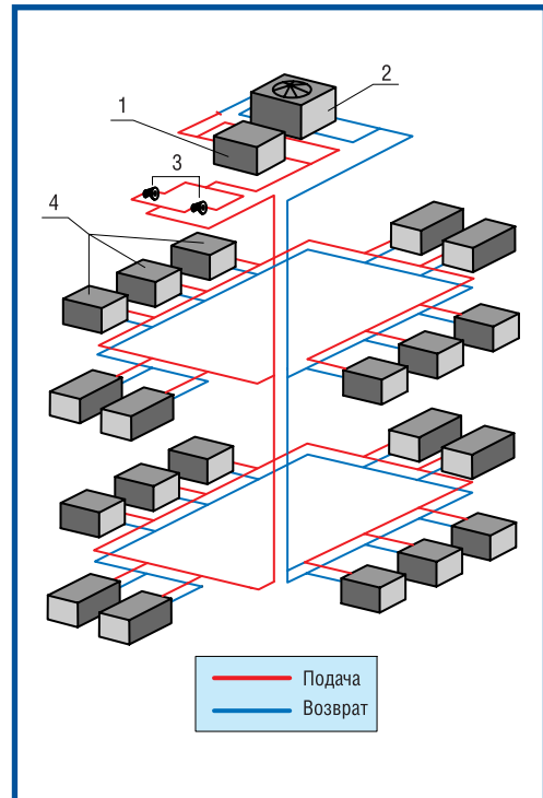
Принципиальная схема системы замкнутого водяного контура с кондиционерами на основе тепловых насосов:
