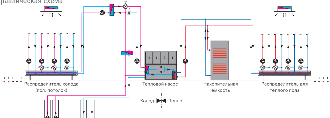
Гидравлическая схема
